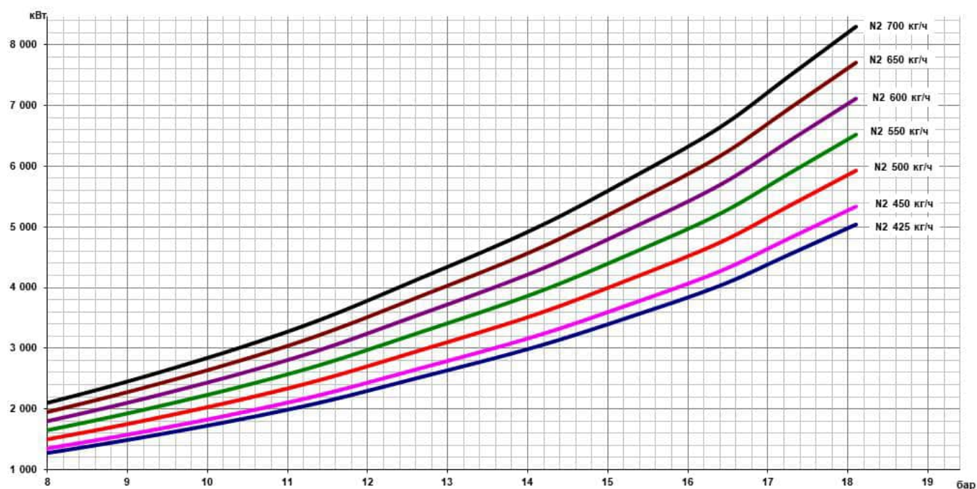
Диаграмма производительности форсунки в зависимости от давления в обратном топливном трубопроводе при давлении насоса 25 бар
